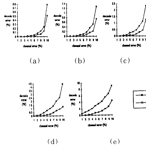
그림 11. Depth별 기존 알고리즘과 제안된 알고리즘의 디코딩 에러 비교 (a) depth = 35 (b) depth = 30 (c) depth = 25 (d) depth = 20 (e) depth = 15
