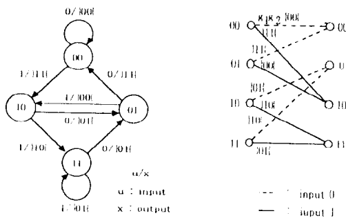
그림 2. 상태도와 trellis 도의 예 (a) 상태도 (b) trellis 도
