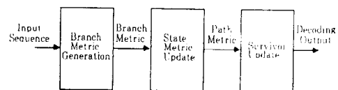
그림 4. Viterbi 디코딩 알고리즘의 하드웨어 블록 구성도
