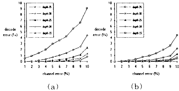
그림 10. 채널에러 vs 디코딩에러
