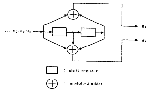
그림 1. R=1/2, K=3인 콘볼루션 인코더
