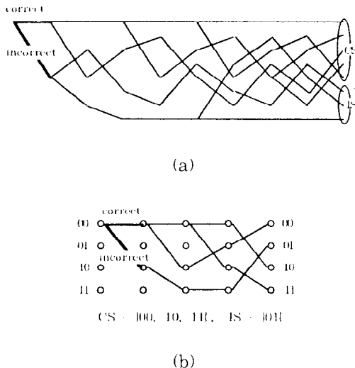
그림 5. Correct subset과 Incorrect subset의 예 (a) 일반예 (b) 특정예
