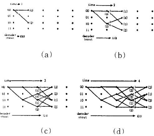
그림 3. Viterbi 알고리즘에서 생존자의 결정과 디코딩 출력의 결정
